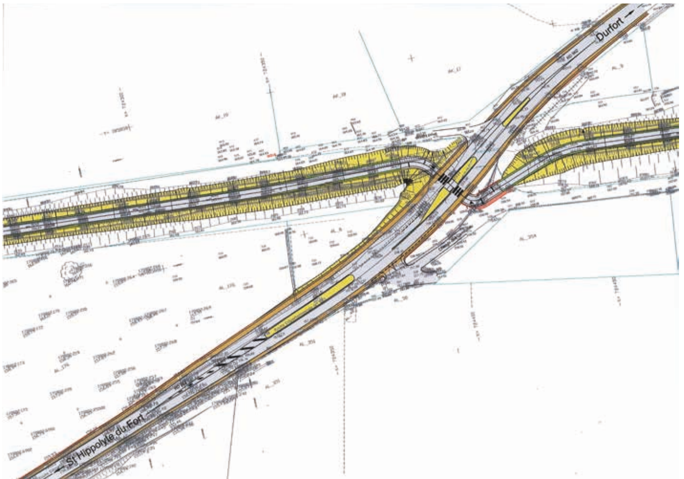
Plan de la sécurisation par le Département du Gard du croisement Voie Verte/D982 au Cambous
